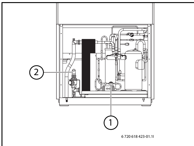
Bild 34 Partikelfilter
