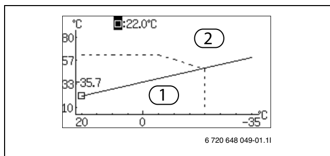
Bild 25 Inställningsfönster Värmekurva (radiator)
