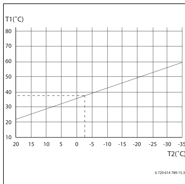
Bild 23 Radiator
