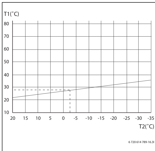
Bild 24 Golv
