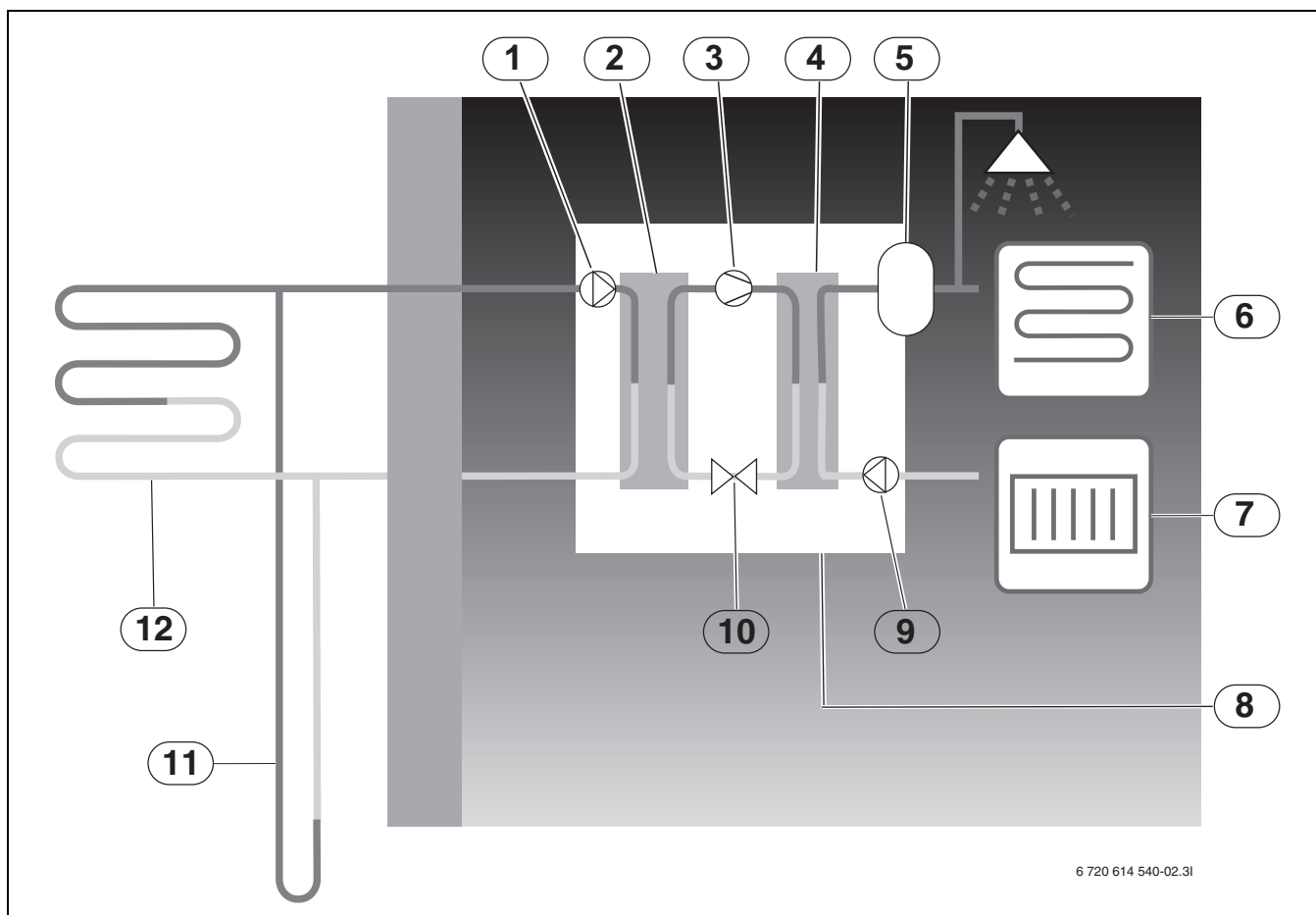
Bild 1 Funktionsbeskrivning
