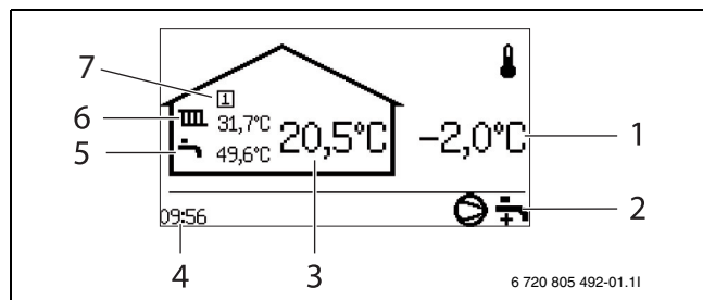
Bild 3 Utgångsläge
