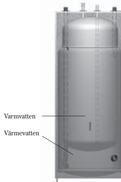
Dubbelmantlad varmvattenberedare
